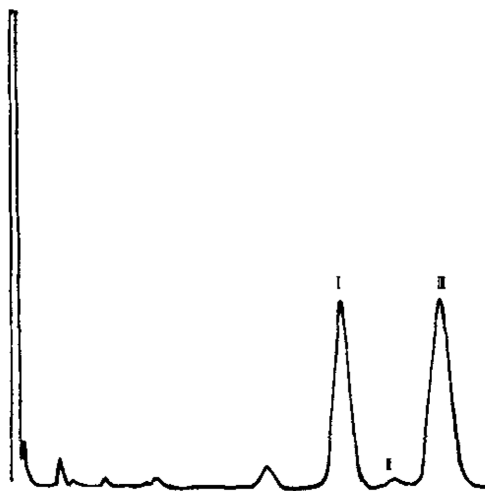
I—邻二苯基苯；II—四氯对苯二甲腈；III—百菌清
