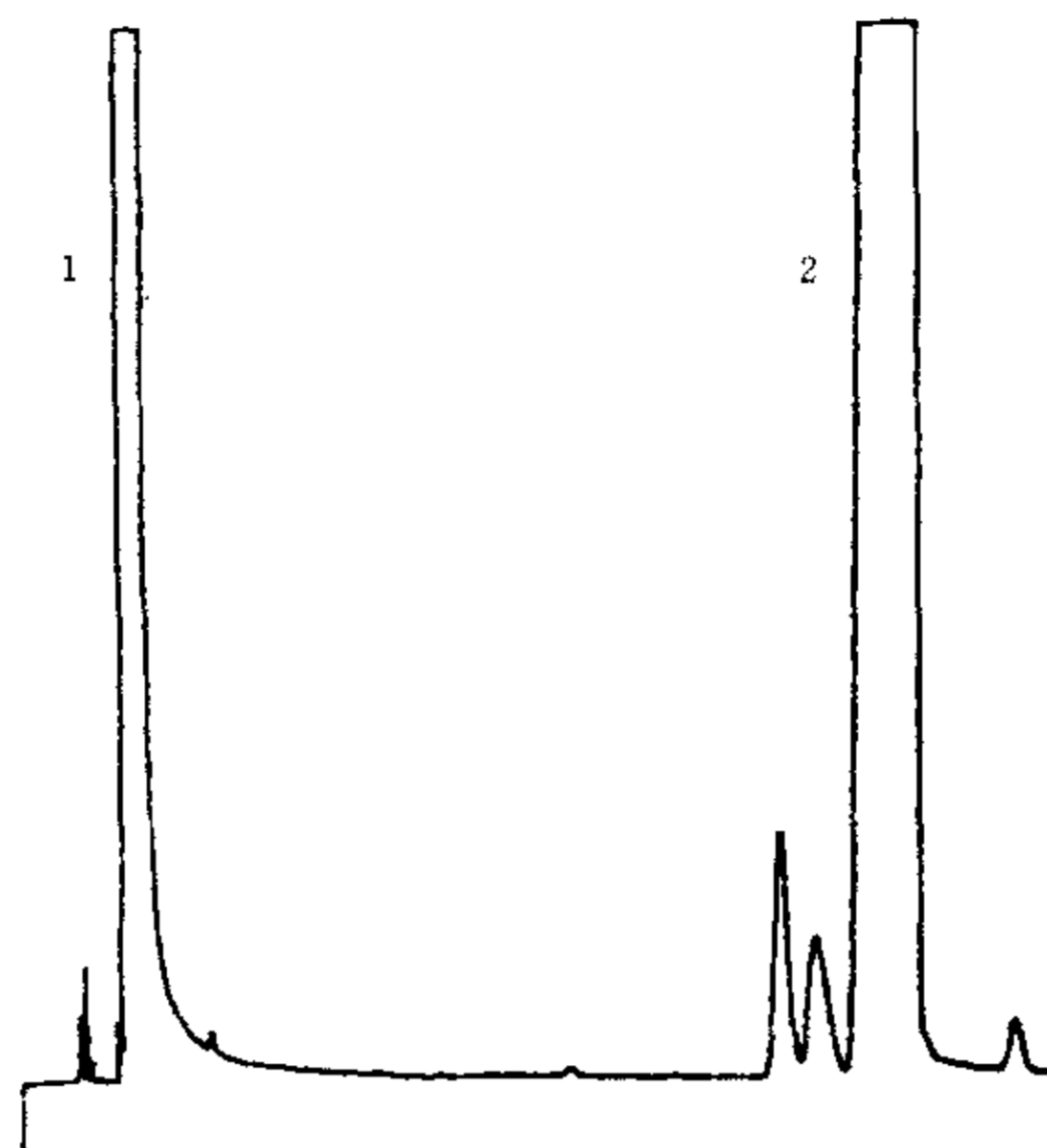
1—六氯苯;2—百菌清
