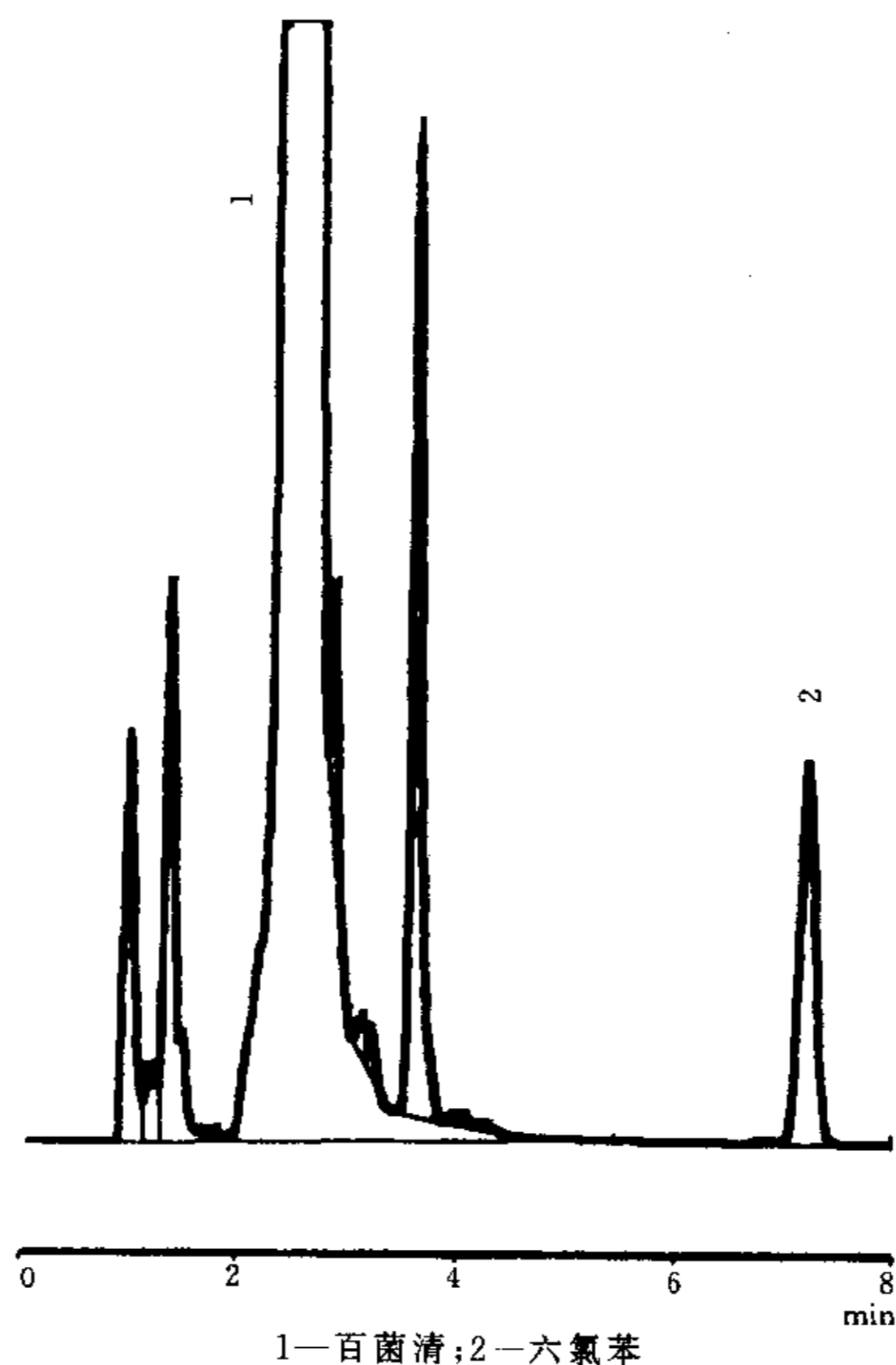
图 2 百草清试样的高效液相色谱图
